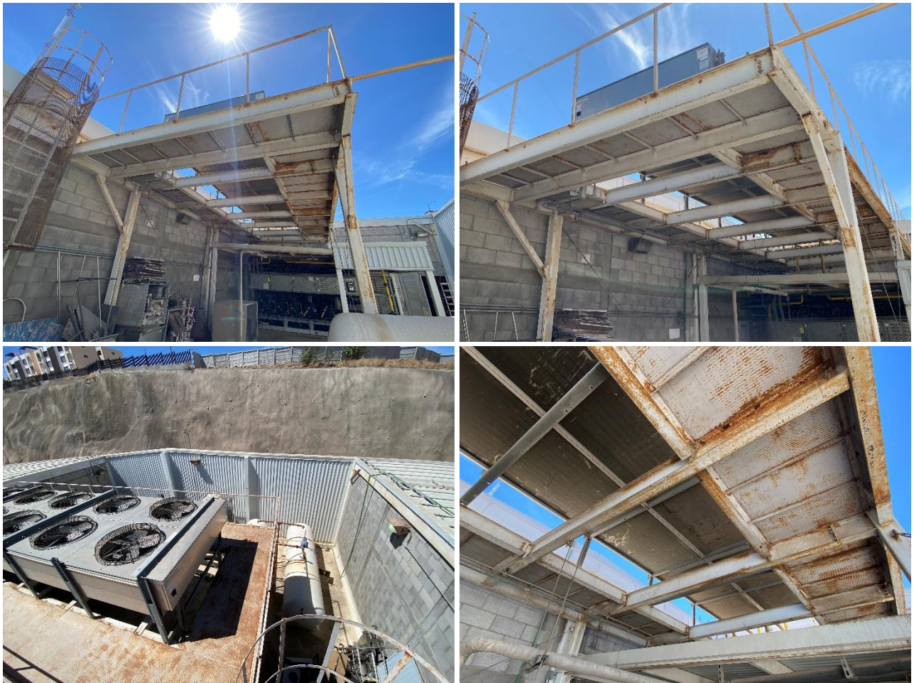
“ELEMENTOS METÁLICOS DE BASE QUE RECIBE CONDENSADORA DE REFRIGERACIÓN”.
